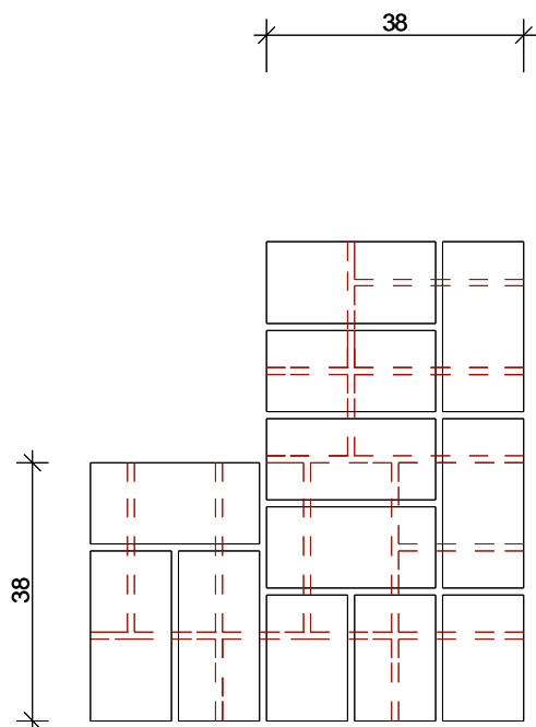
Másfél téglák vastag falsarok
