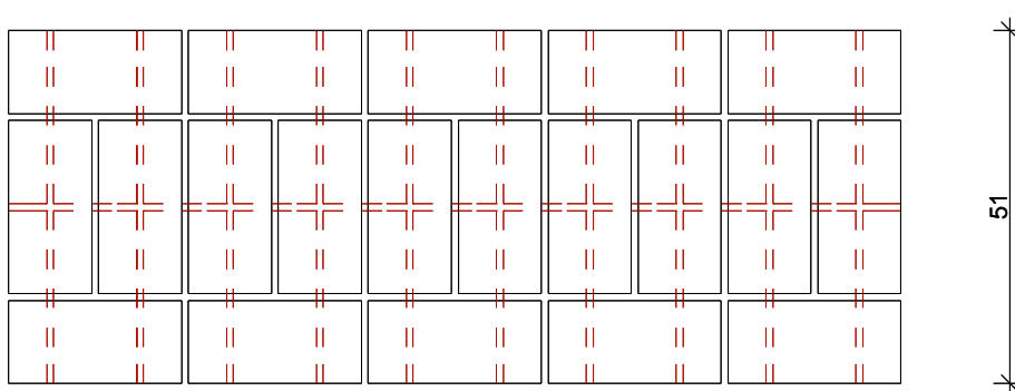
Két téglá vastag fal
