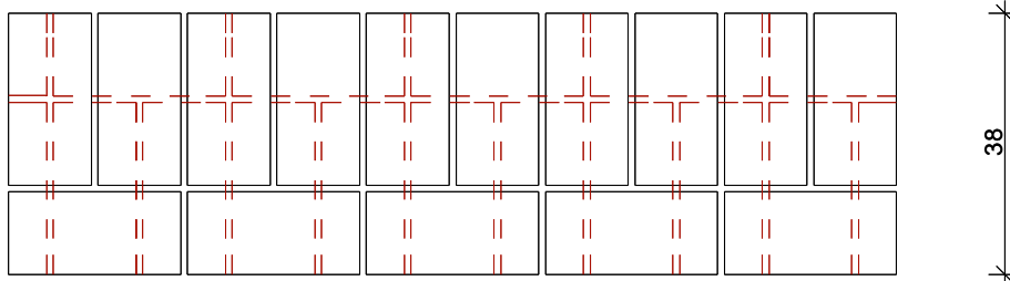
Két téglá vastag fal
