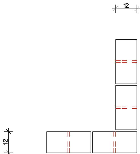
Másfél téglák vastag falsarok
