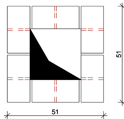
51 x 51 cm kéménypillér
