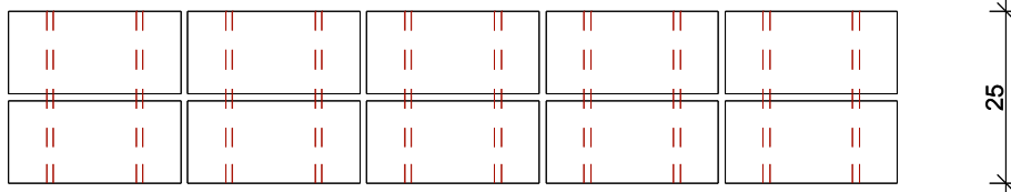
Másfél téglá vastag fal
