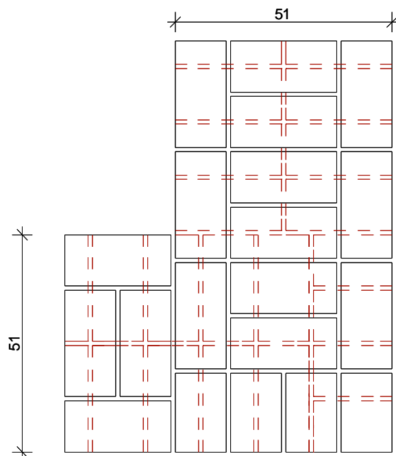
Két téglák vastag falsarok
